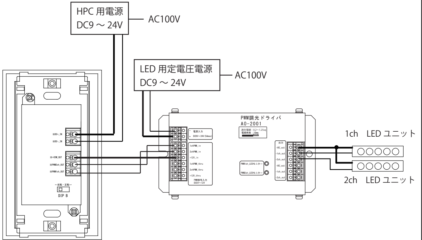
2ch PWM ライトコントローラ HPC-2101
